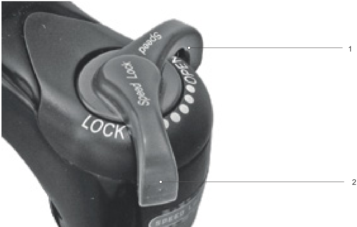
Figura 127: Amortiguador de niveles de presión Suntour en posición abierta (1) y cerrada (2)
