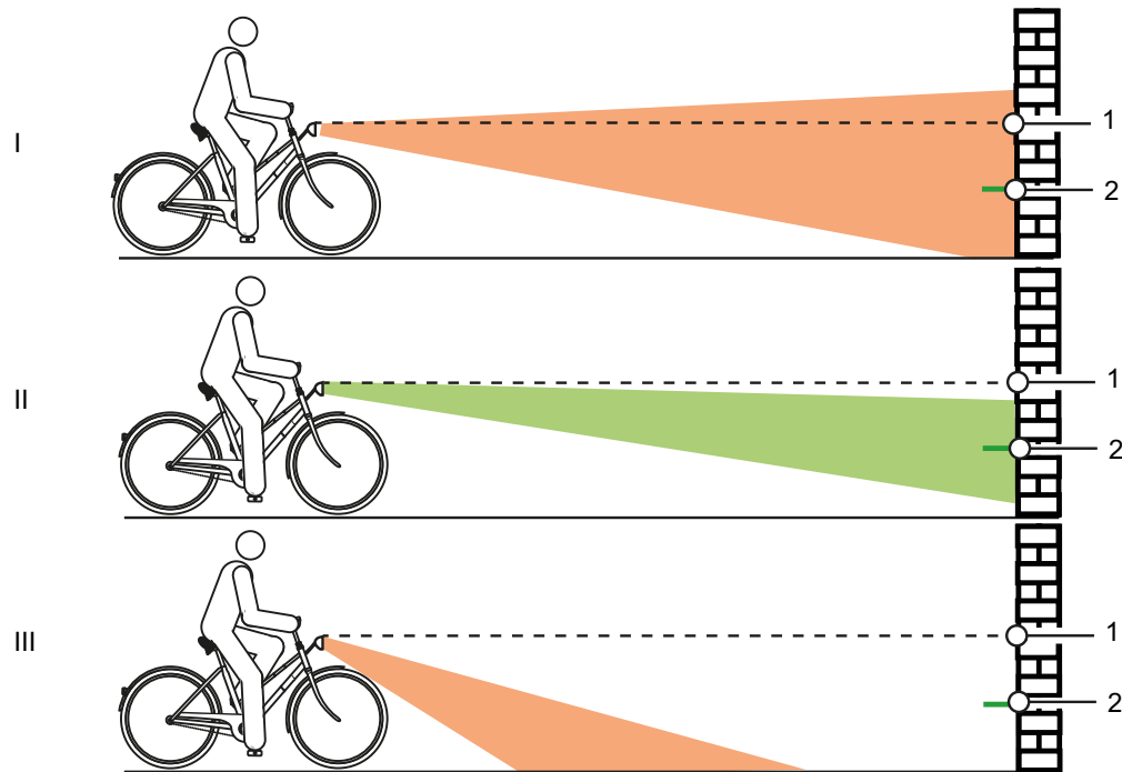
Figura 138: Luz ajustada demasiado alta (1), correctamente (2) y demasiado baja (3)
