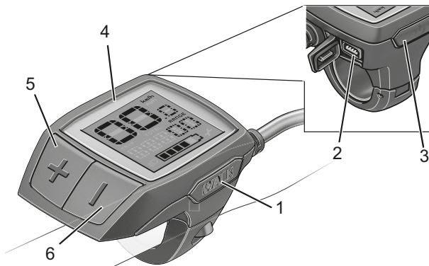
Figura 37: Estructura del ordenador de a bordo BOSCH Purion
