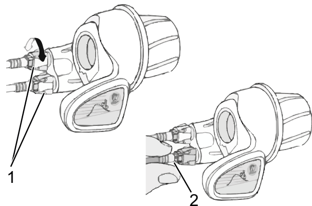
Figura 144: Puño giratorio con casquillos de ajuste (1) y holgura del cambio de marchas (2)
