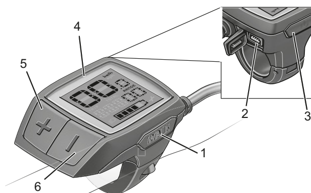
Figura 123: Estructura del ordenador de a bordo BOSCH Purion
