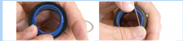
Figura 197: Inserción y fijación del rascador
