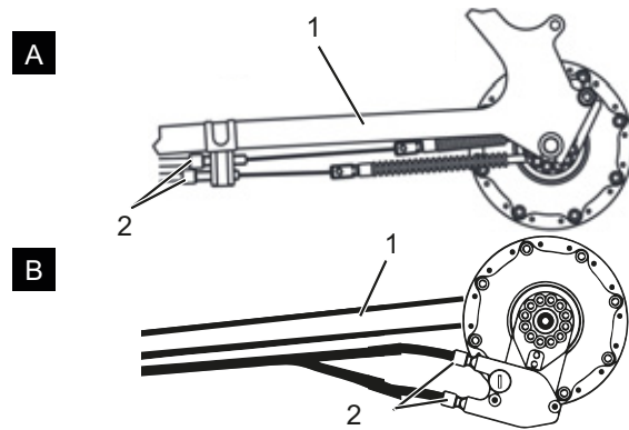
Figura 143: Casquillos de ajuste (2) en dos versiones alternativas (A y B) de un cambio de marchas accionado por cable de accionamiento, de dos cables en la vaina (1)
