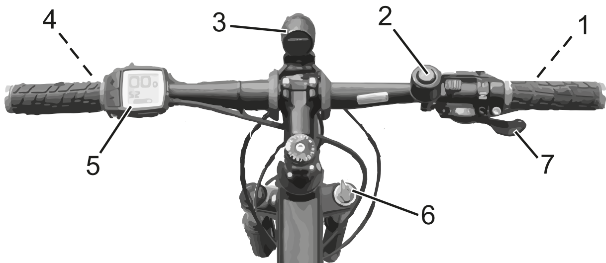
Figura 36: Vista detallada del manillar desde la posición de asiento, ejemplo
