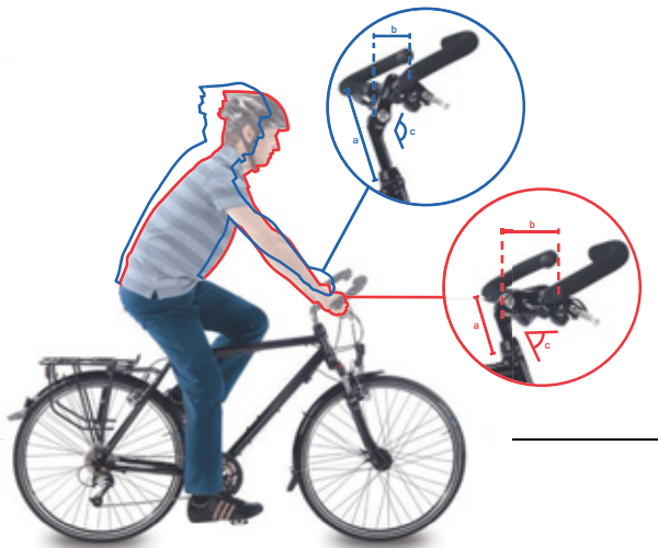
Figura 95: Posición de la bicicleta de ciudad (azul) y la bicicleta de trekking (rojo) mediante la modificación angular
