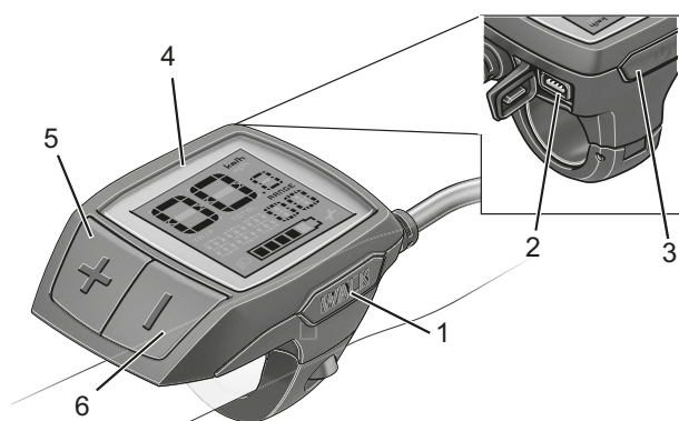
Figura 110: Estructura del ordenador de a bordo BOSCH Purion
