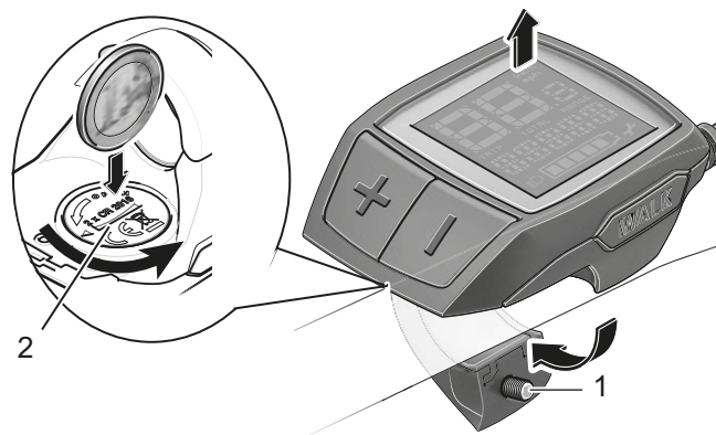
Figura 124: Ordenador de a bordo con tornillo de fijación (1) y tapa del compartimento de la batería (2)
