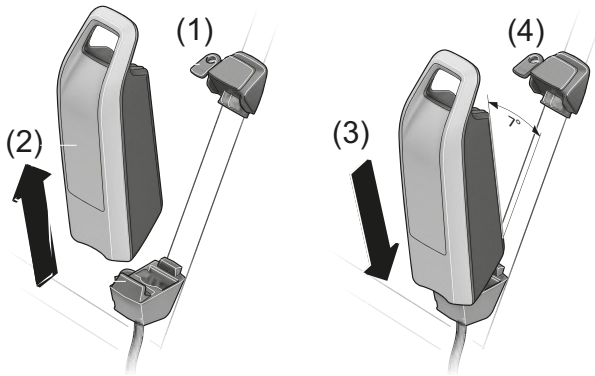
Figura 118: Extracción e inserción de la batería en el cuadro
